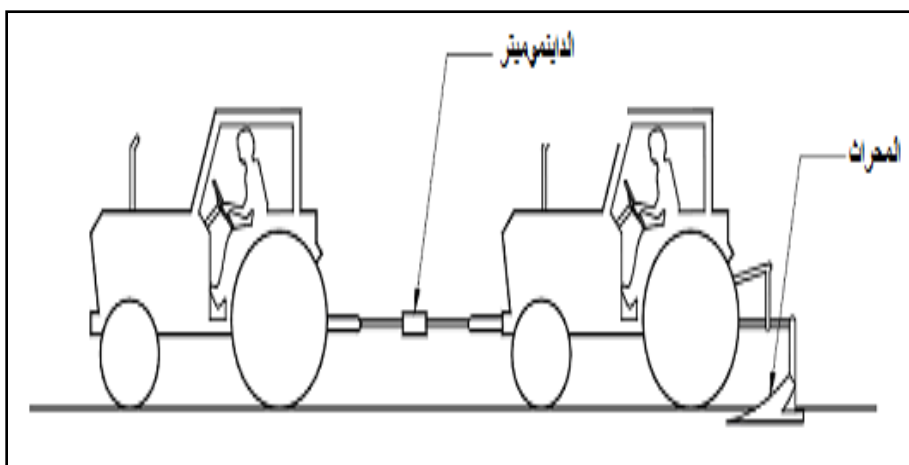
الشكل (2): طريقة قياس قوة السحب للمحراث تحت التربة ثنائي السلاح
